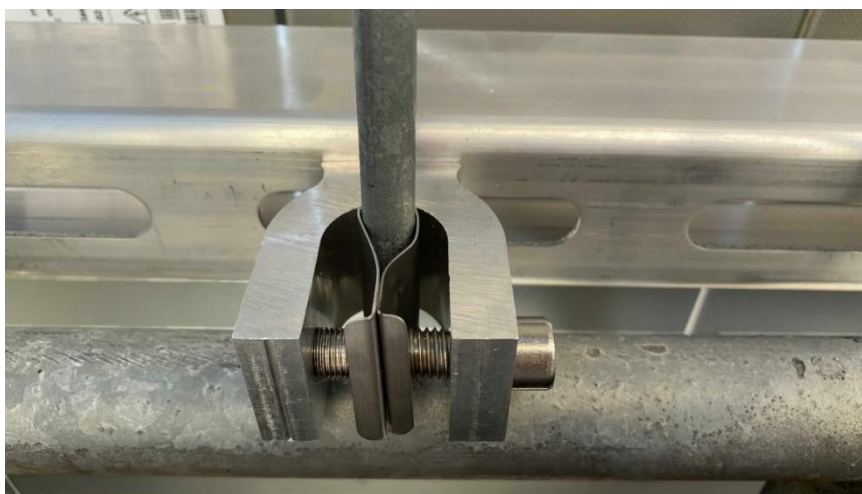
Abb. 8/Spezialklappe an Rundstab
