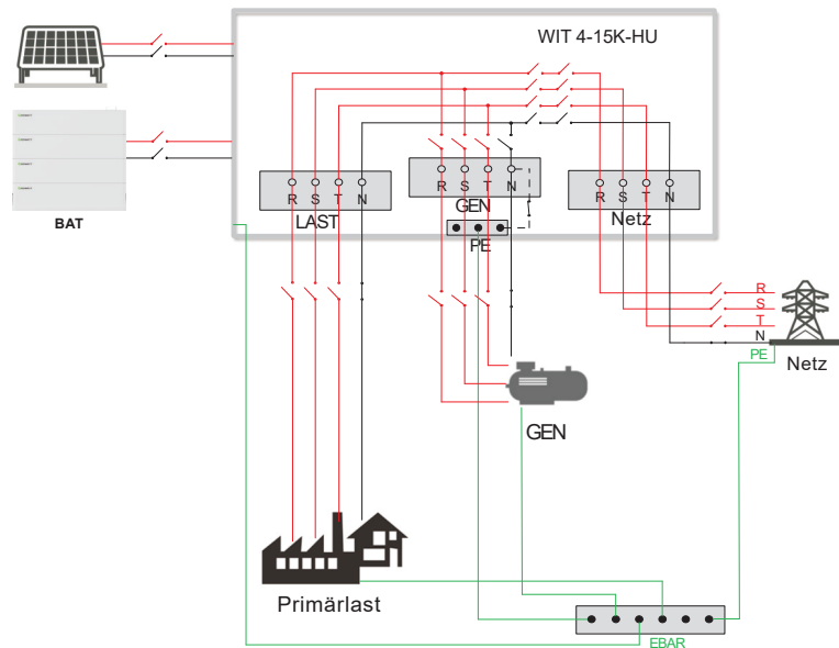
(b) Schaltplan für andere Regionen
