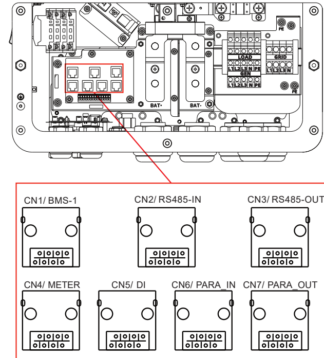
Abb 6.17 Kommunikationsnetzwerkanschluss
