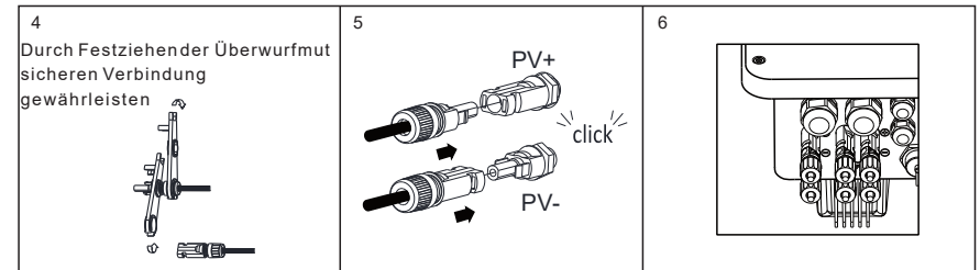
Abb 6.13 PV-Anschlussklemmen
