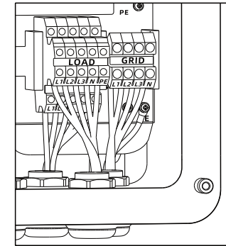
Abb 6.11 AC-Anschlussklemmen und Schaltplan
